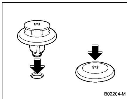
Clips des Typs C
