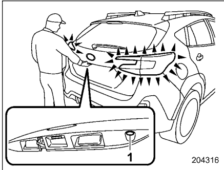
1 Heckklappenverriegelungstaste
