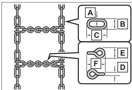
Seitliche Kette:
