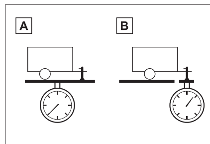
A Gesamtgewicht des Anhängers
